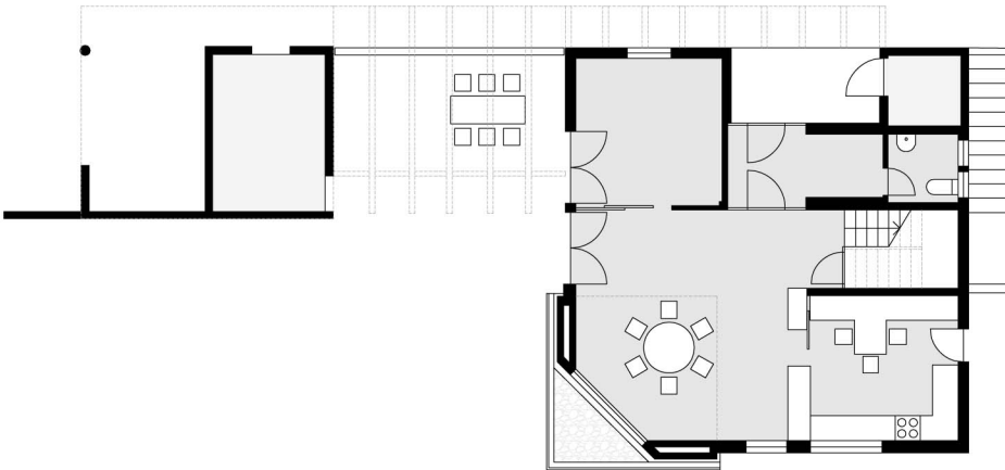
ERDGESCHOSS
