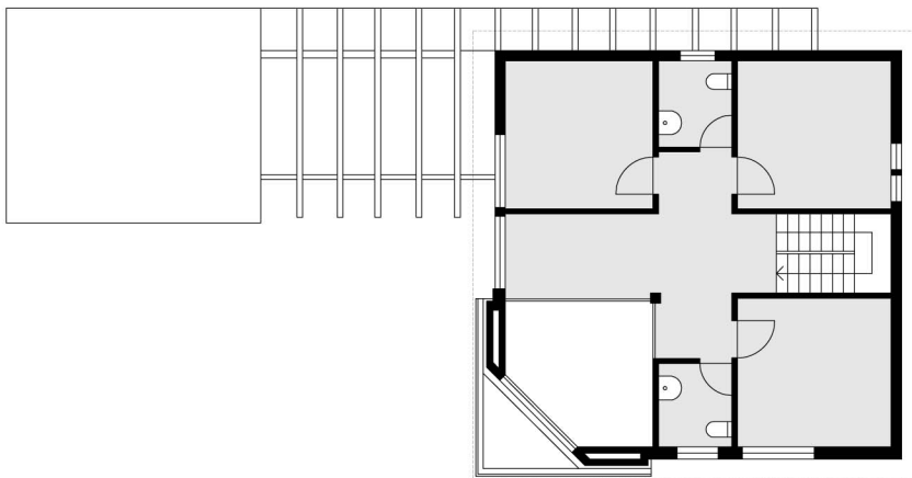
OBERGESCHOSS
